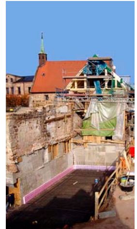
Unterfangung Stadtmauer und Giebel Altbau; Bodenplatte Anbau
